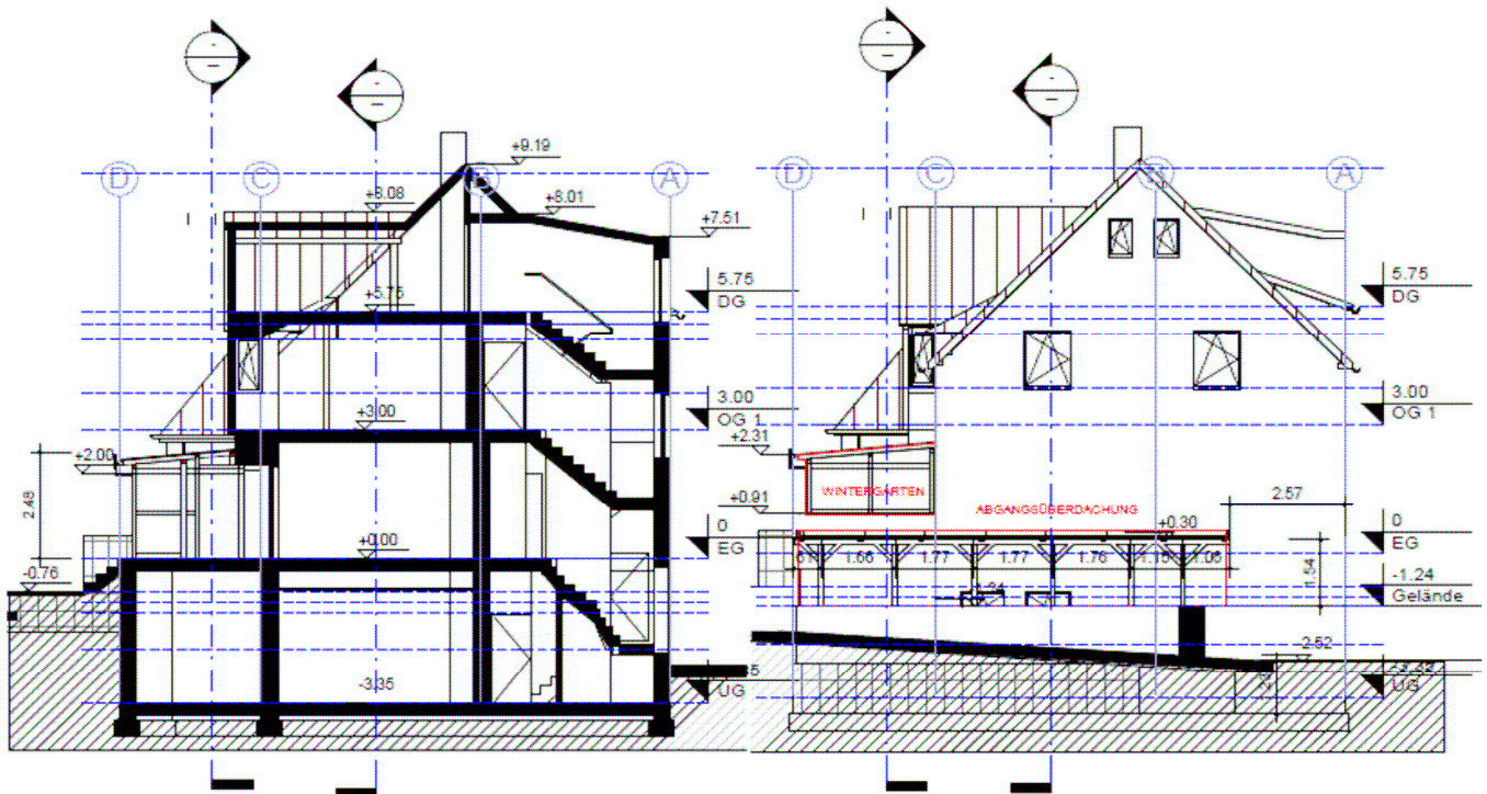
2 Süd 1 : 100
